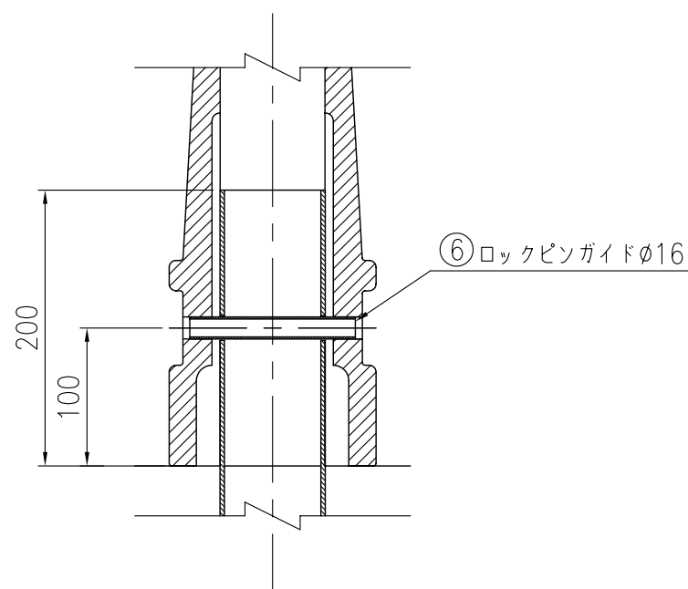
下部断面詳細図
