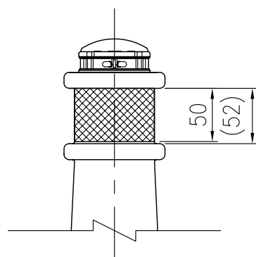
反射シート貼付部詳細
