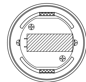
SLキャップ80 S=1/2
