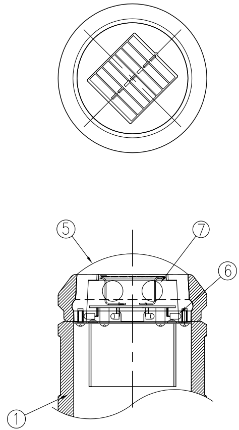
自発光頭部詳細
