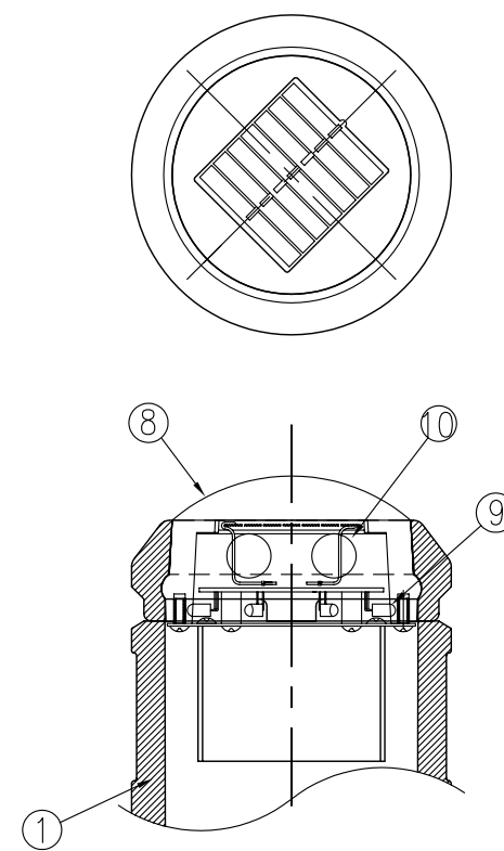
自発光頭部詳細
