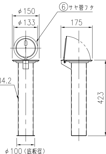
サヤ管詳細図
