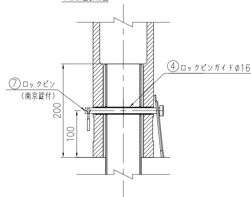
下部断面詳細図
