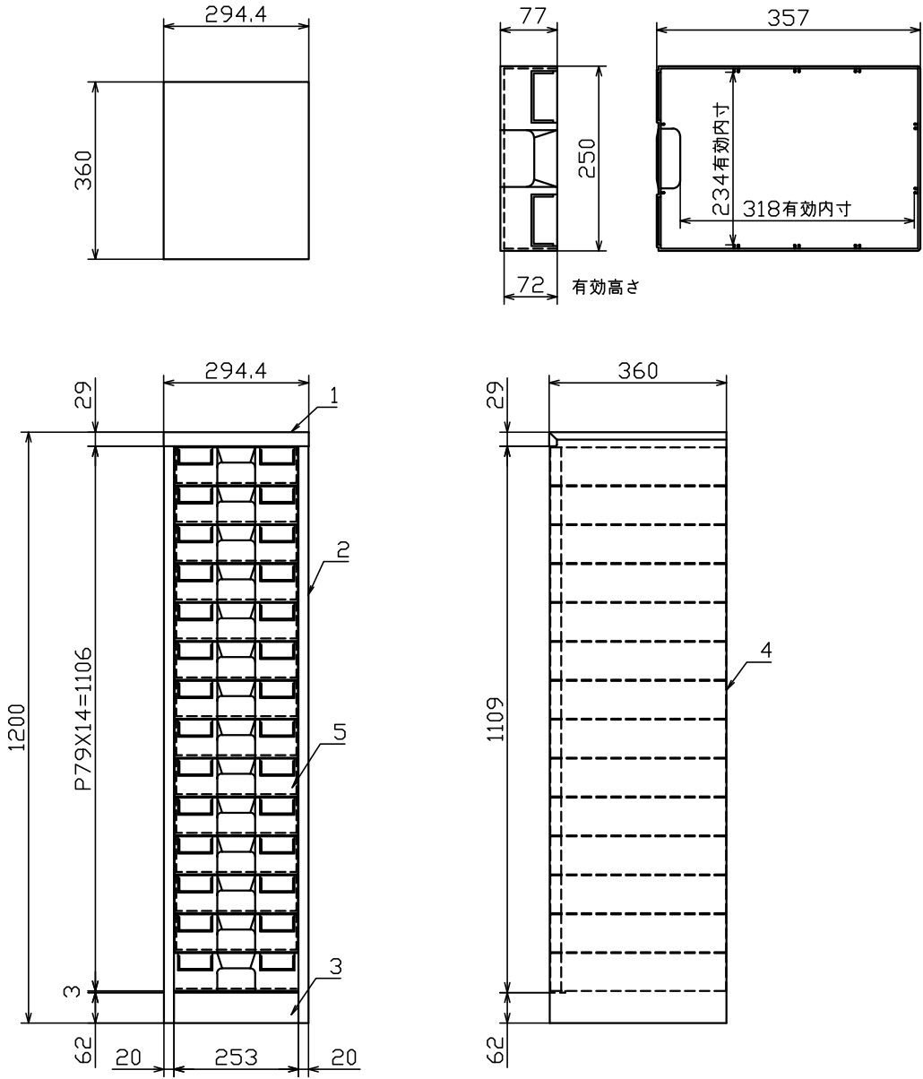
引出詳細図
