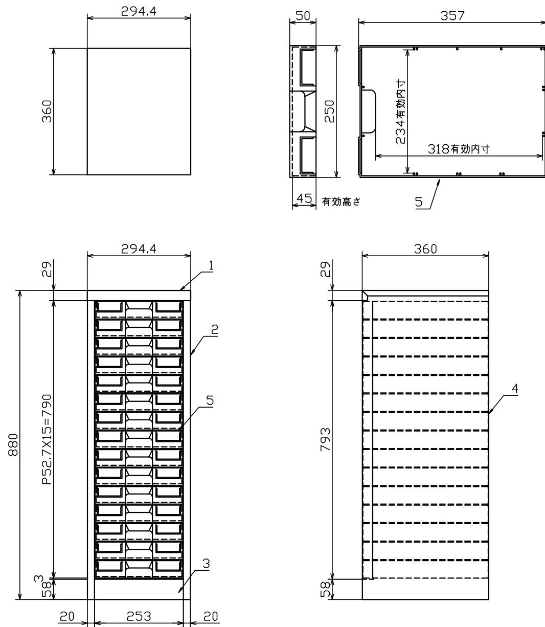
引出詳細図
