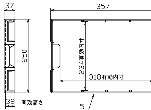
引出詳細図
