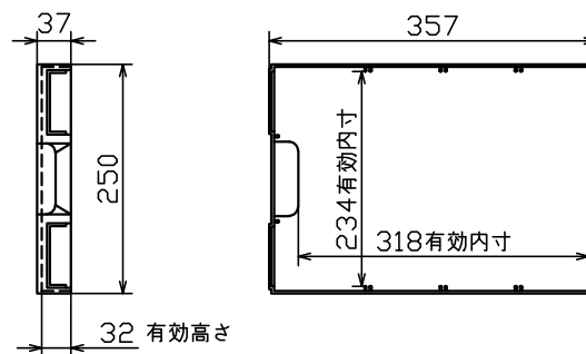
引出詳細図
