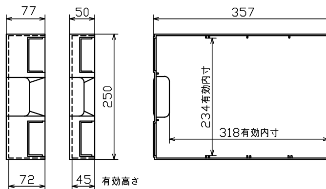
引出詳細図
