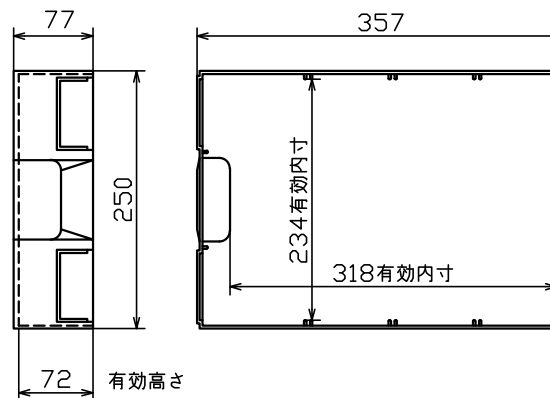
引出詳細図
