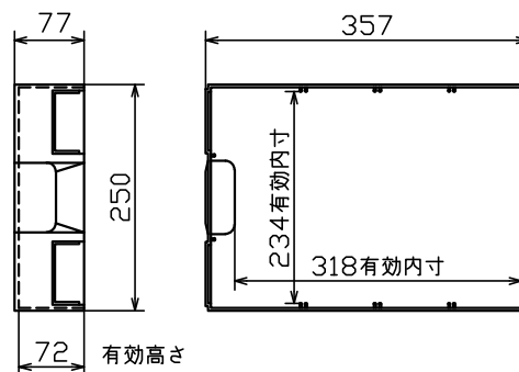
引出詳細図
