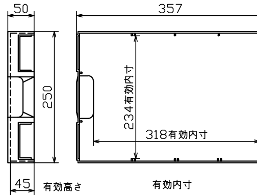
引出詳細図
