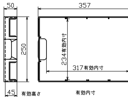
引出詳細図
