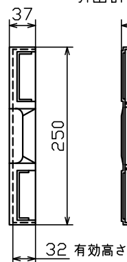
引出詳細図
