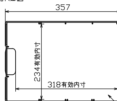
引出詳細図
