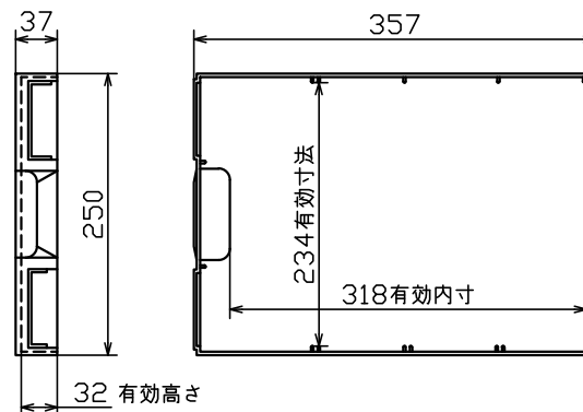
引出詳細図
