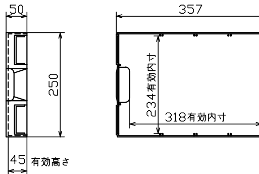
引出詳細図
