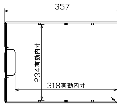
引出詳細図
