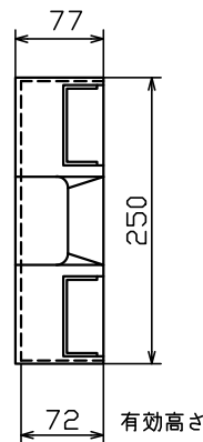
引出詳細図
