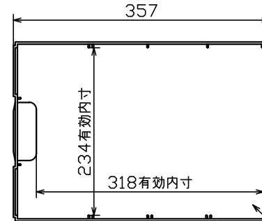
引出詳細図
