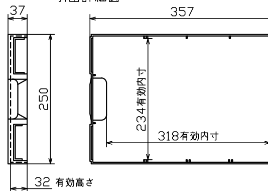
引出詳細図
