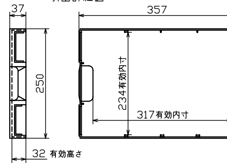
引出詳細図
