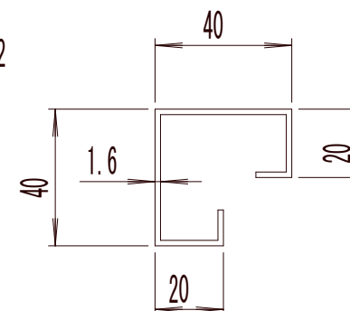
脚断面図 S=1:2
