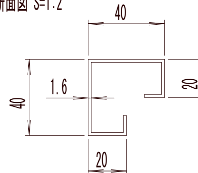
脚断面図 S=1:2
