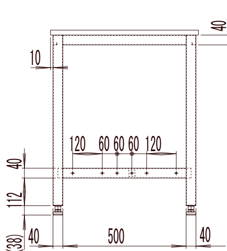
脚断面図 S=1:2
