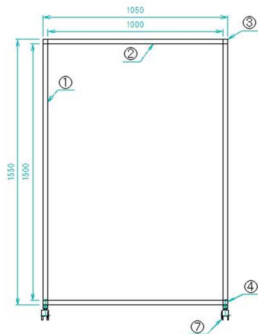
正面図
