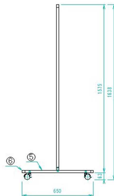
側面図
