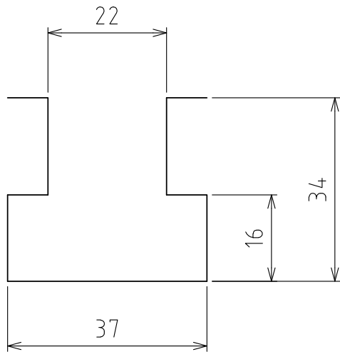
T溝寸法
