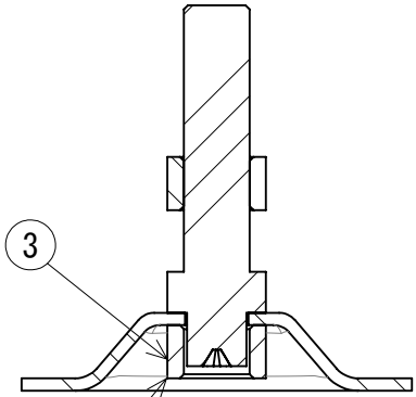
ナット圧入 断面図 A-A
