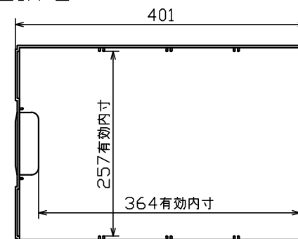
引出詳細図
