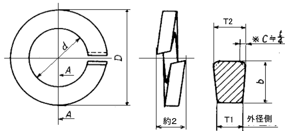
断面 A-A
