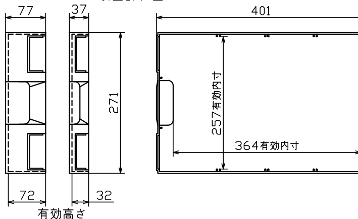
引出詳細図
