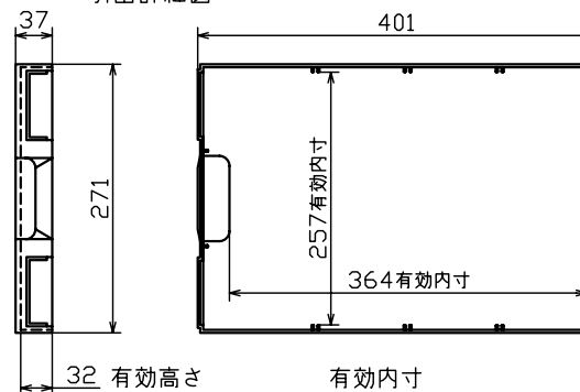
引出詳細図
