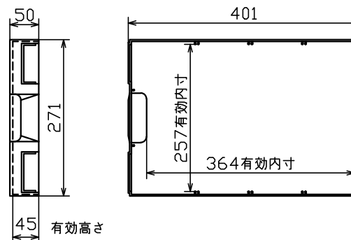
引出詳細図
