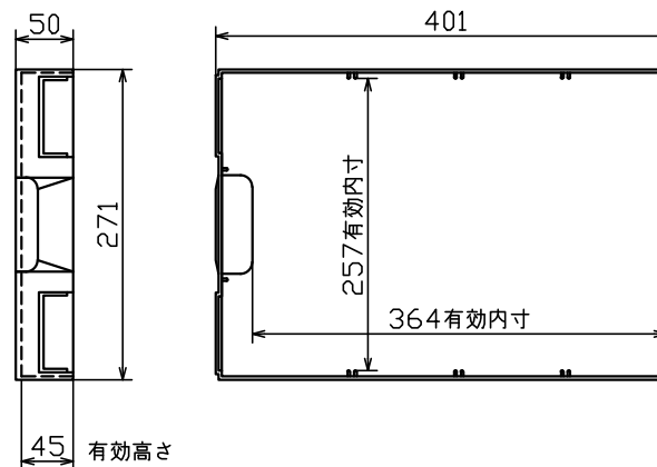
引出詳細図
