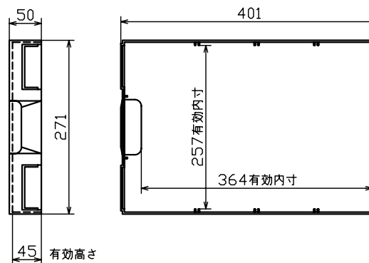
引出詳細図
