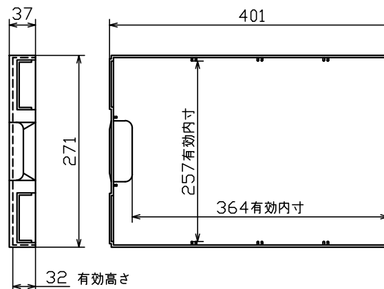
引出詳細図
