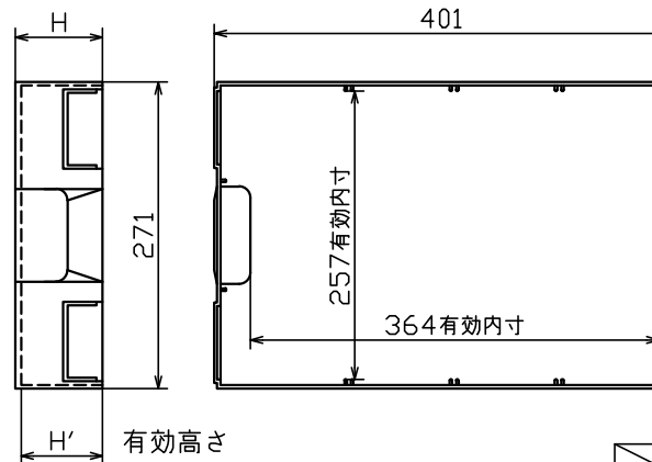
引出詳細図
