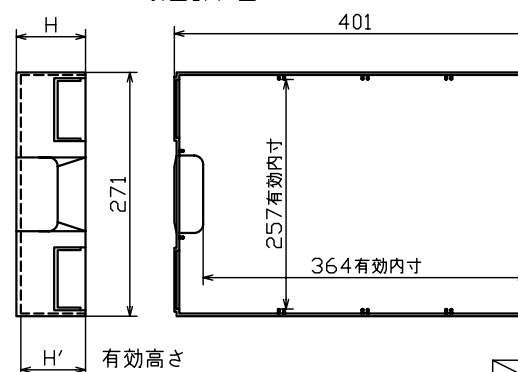
引出詳細図
