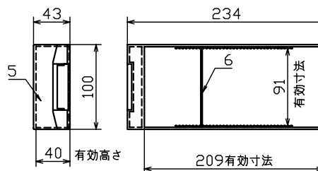
引出詳細図
