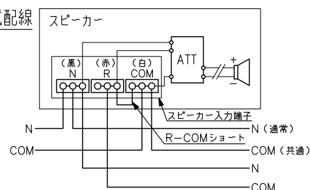
回路図
