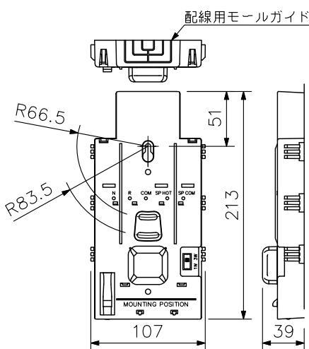
スピーカーコンセント (付属) (縮尺: 1/5)
