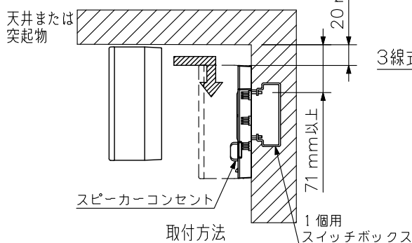
スピーカーコンセント (付属) (縮尺: 1/5)
