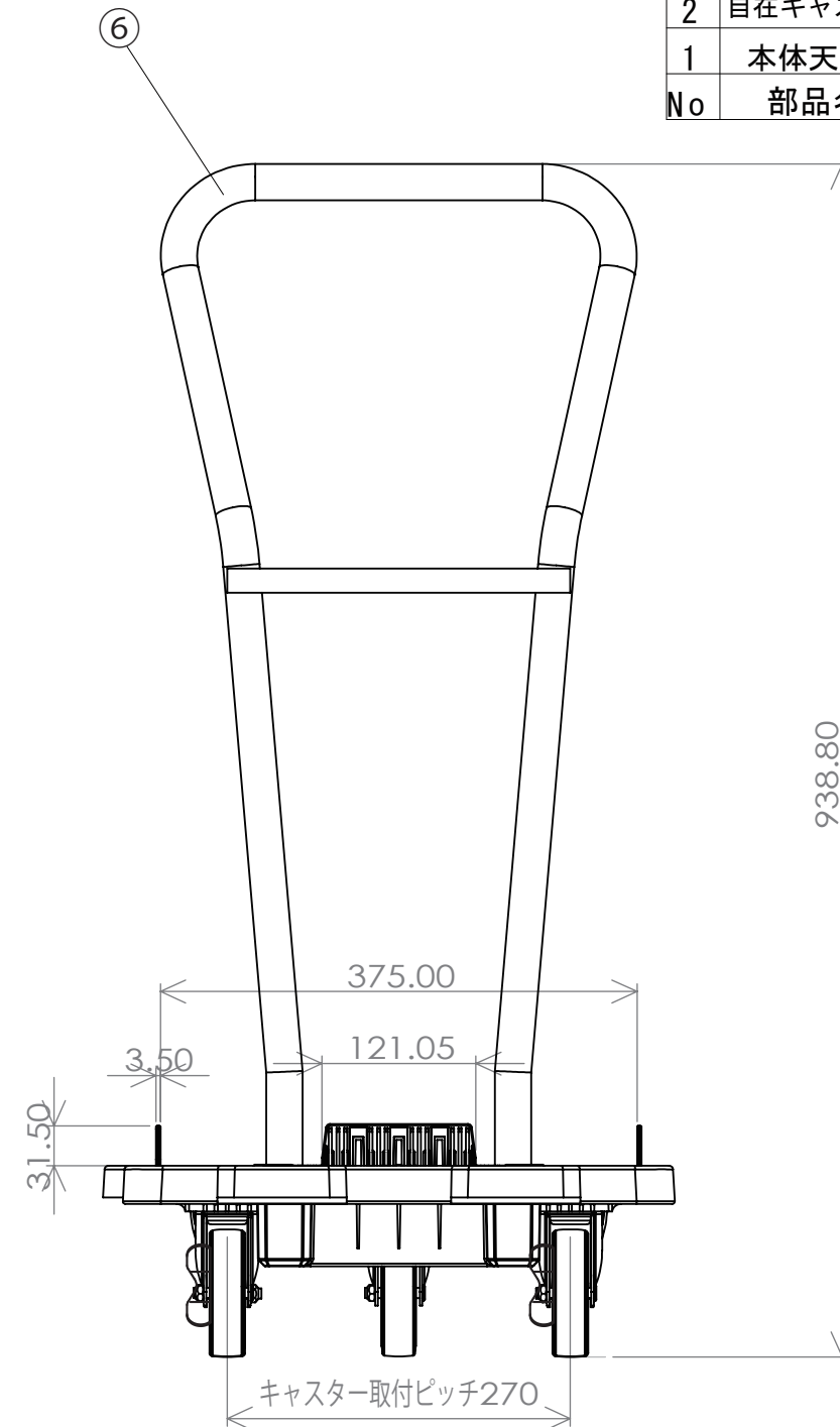
裏面キャスター取付部
