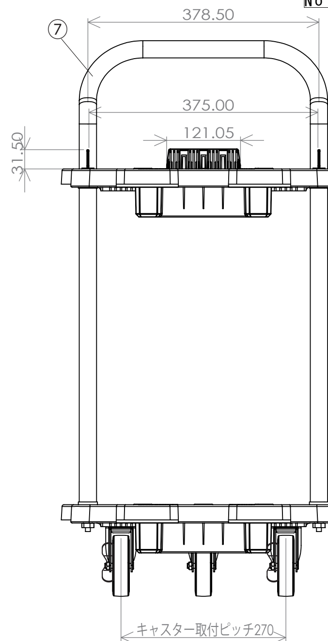
裏面キャスター取付部
