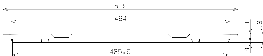
正 面 図
