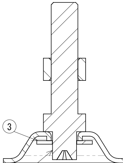
断面図 A-A
