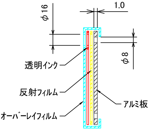
断面A-A
