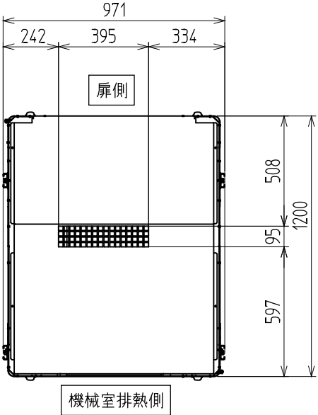
A-A 吸気口位置図
