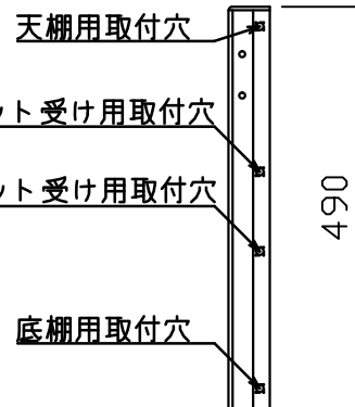
支柱取付穴詳細図
