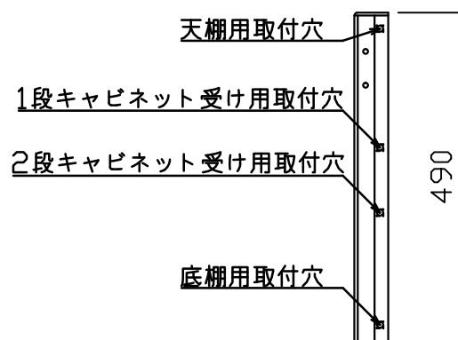
支柱取付穴詳細図
