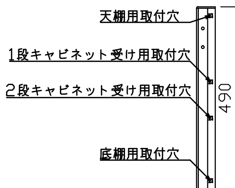
支柱取付穴詳細図
