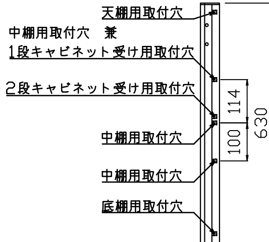
支柱取付穴詳細図
