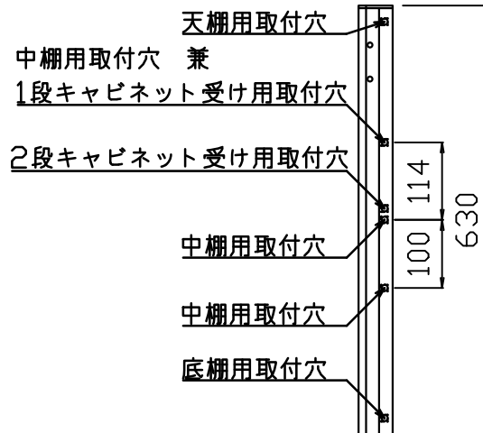
支柱取付穴詳細図
