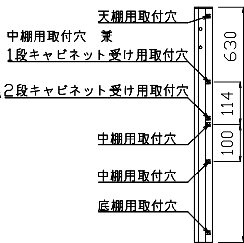
支柱取付穴詳細図
