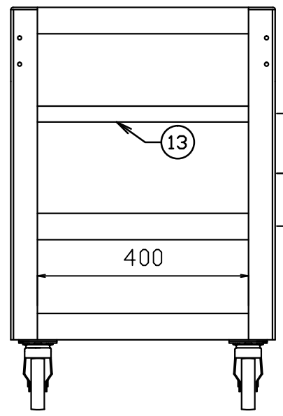
支柱取付穴詳細図
