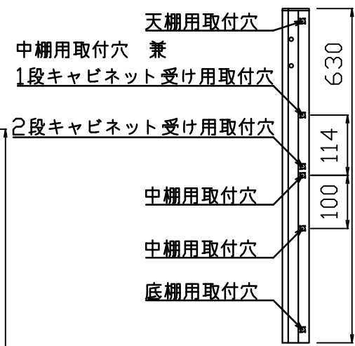
支柱取付穴詳細図
